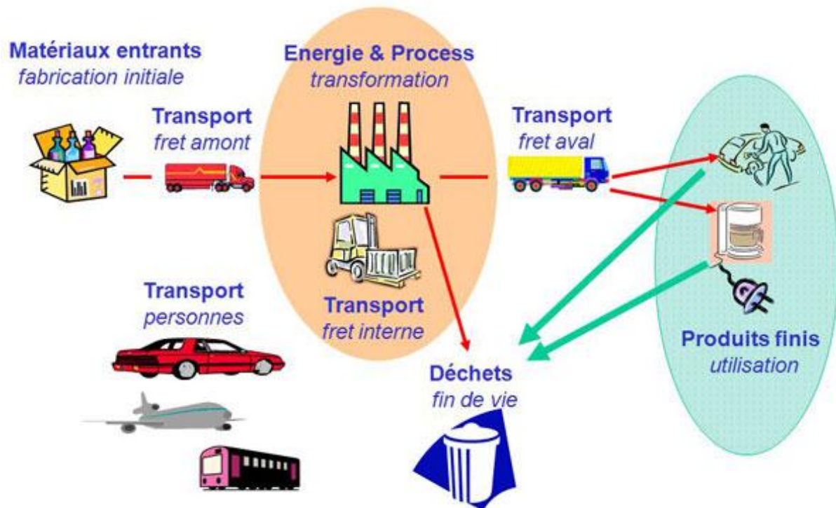
Figure 1 : les principaux postes d'émission de CO 2
